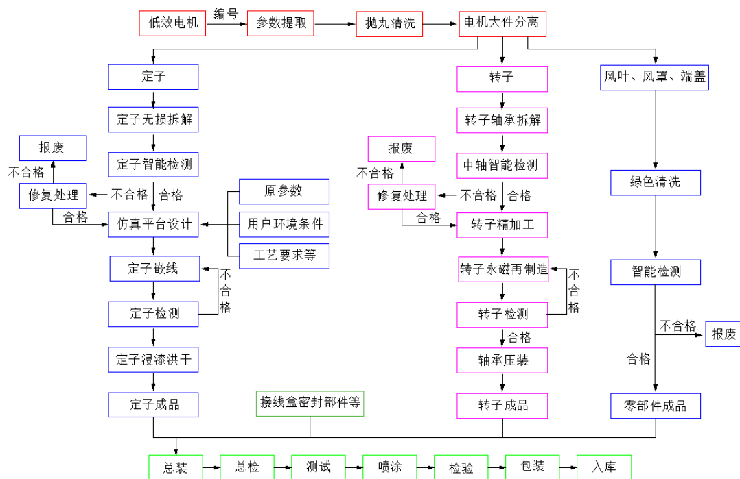
低效电机永磁化再制造工艺流程图
